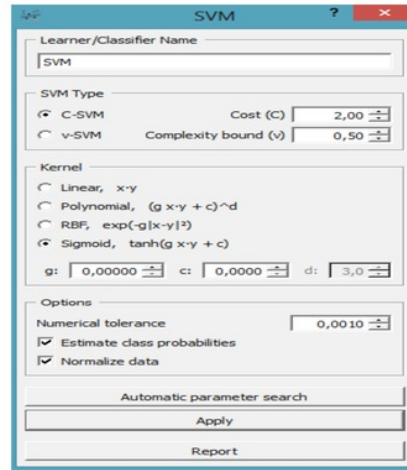
Gambar 4. Paramater metode SVM
