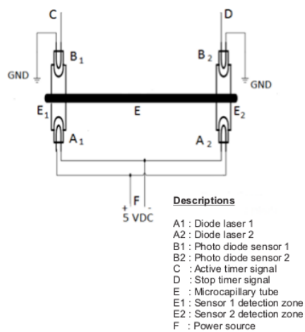
Figure 1. Digital microcapillary. (Source: Rasyid A. Modifikasi Mikrokapiler Digital untuk Mengukur Nilai Viskositas Darah dan Viskositas Plasma. Kementerian Hukum dan Hak Asasi Manusia R.I. Direktorat Jenderal Hak Kekayaan Intelektual Direktorat Paten P00201300222, Mar. 2013)
